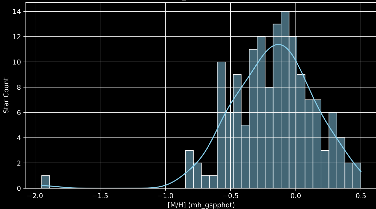
APOGEE DR17 Field: [282-29-O_TESS [M/H] (mh_gspphot) (n= 148)
