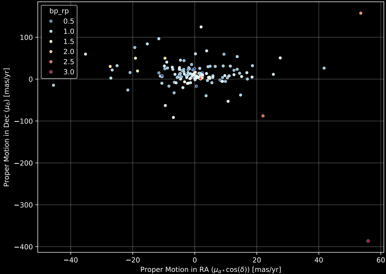
APOGEE DR17 Field: [282-29-O_TESS] Proper Motion Diagram (n= 149)
