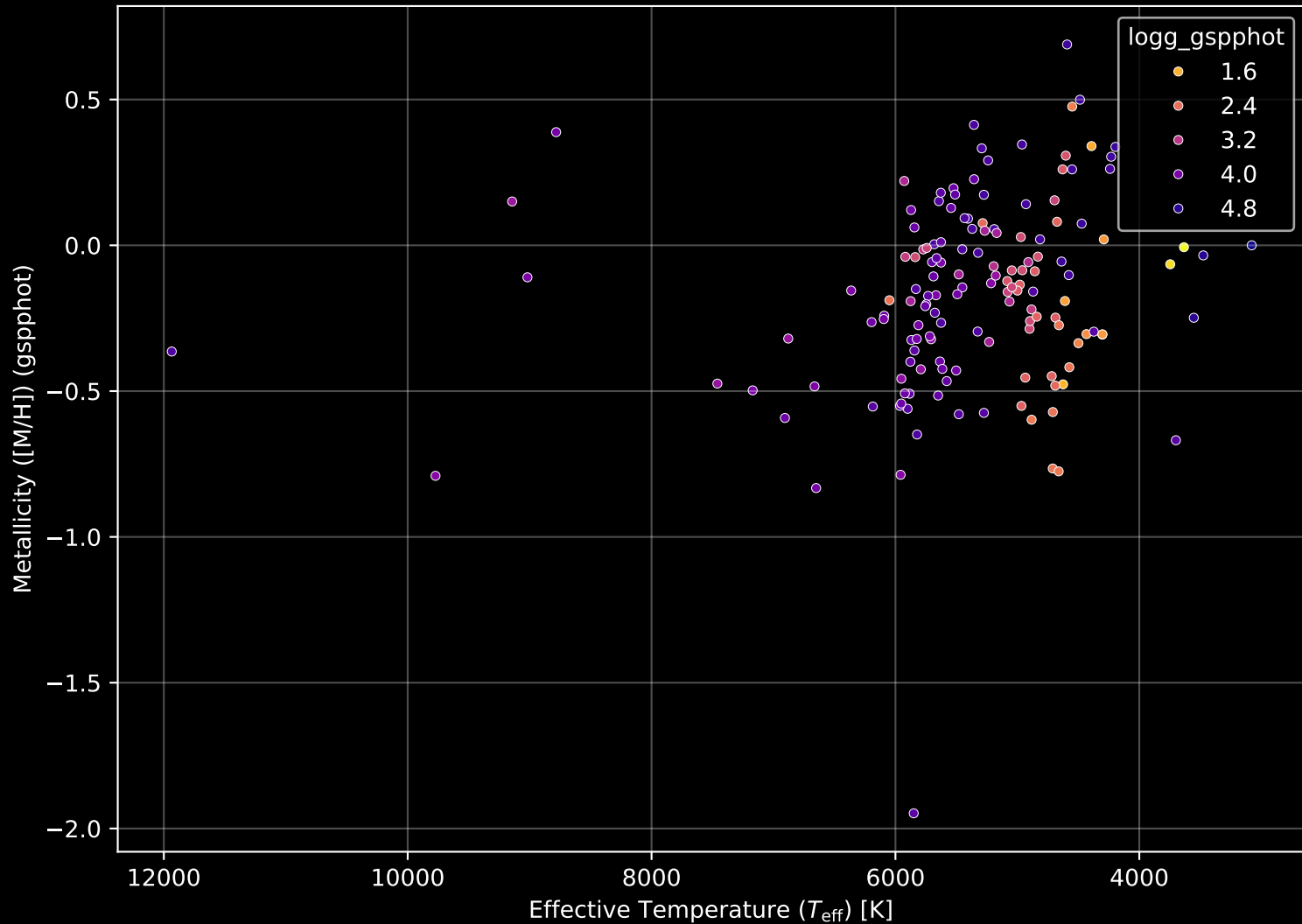
APOGEE DR17 Field: [282-29-O_TESS] Stellar Population Parameters (n= 149)
