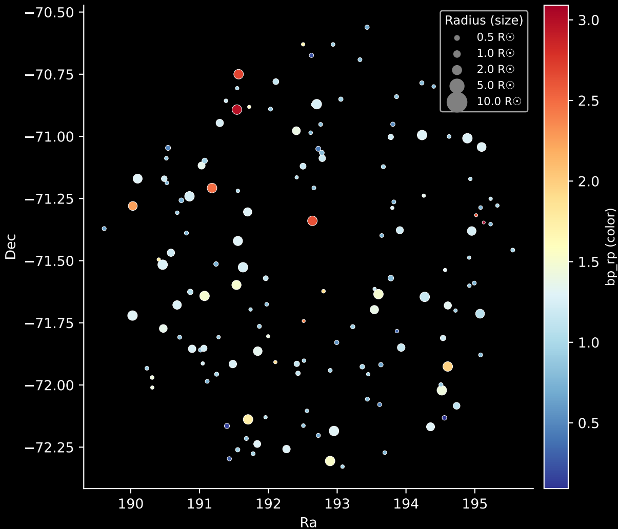
APOGEE DR17 Field: [282-29-O_TESS] Stars: 149
